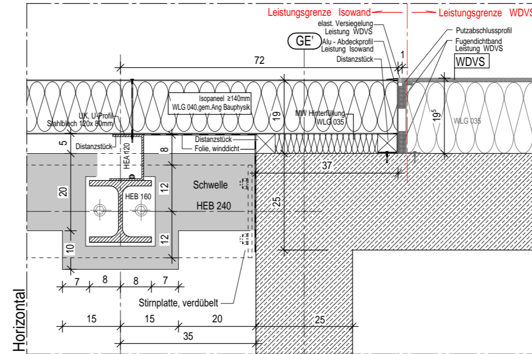
DETAIL 3 M. 1:10
