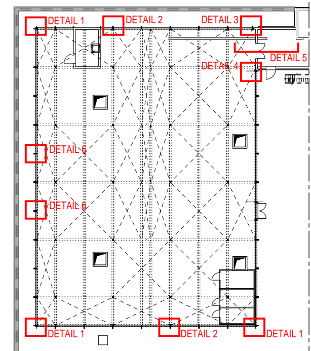
ÜBERSICHTSPLAN
