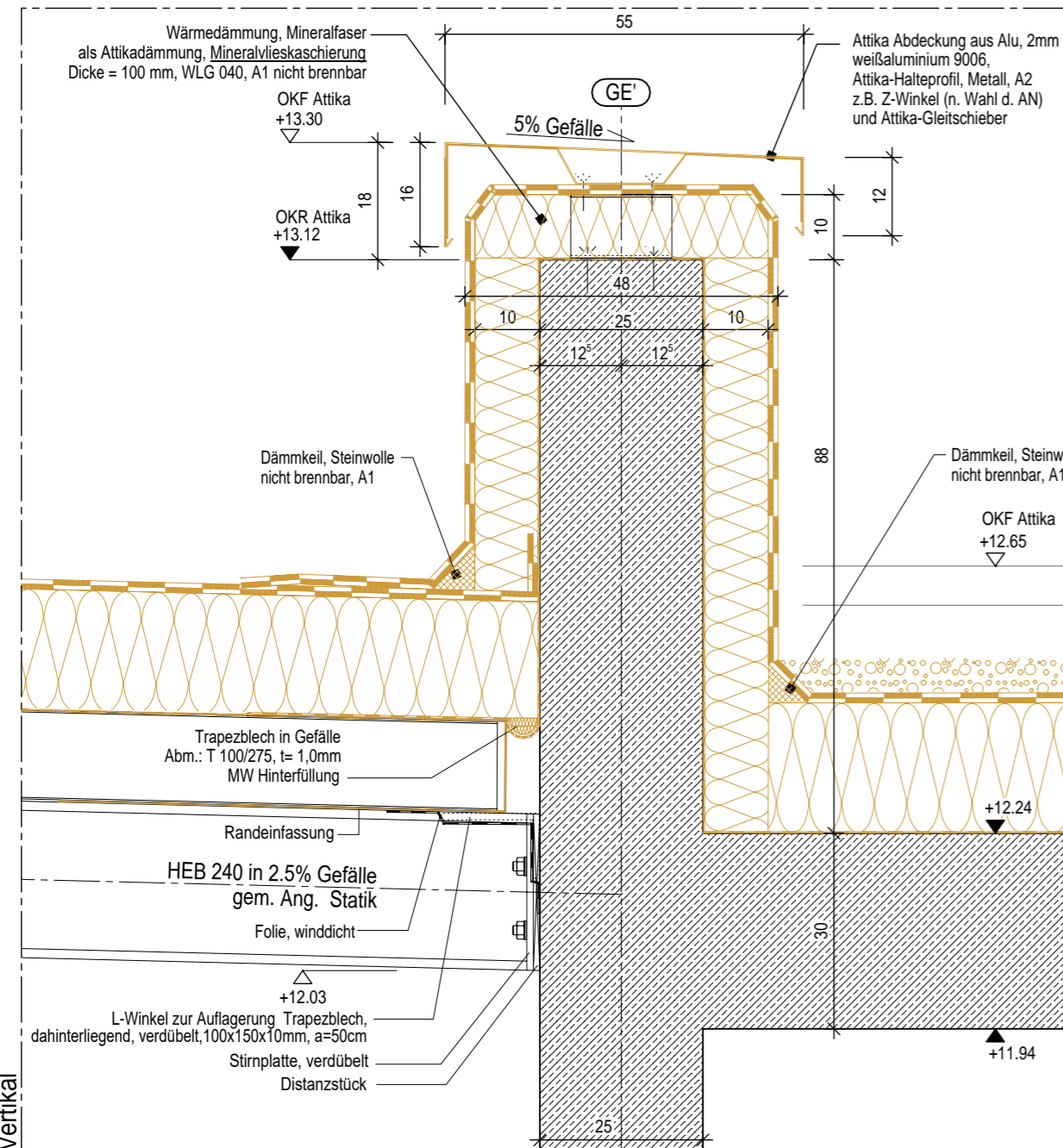
DETAIL 5 M. 1:10
