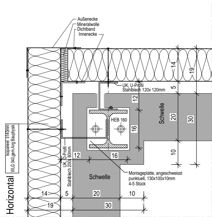
DETAIL 1 M. 1:10
