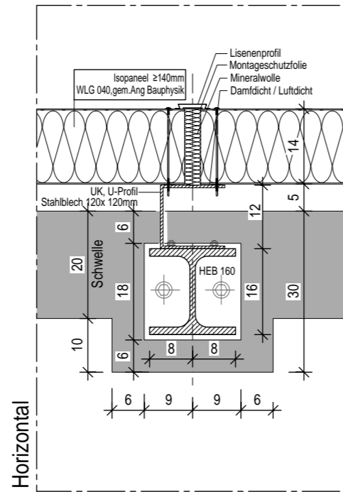
DETAIL 2 M. 1:10
